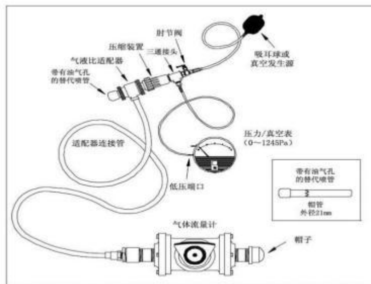
图C.4 气液比适配器泄漏检测装置安装示意图
