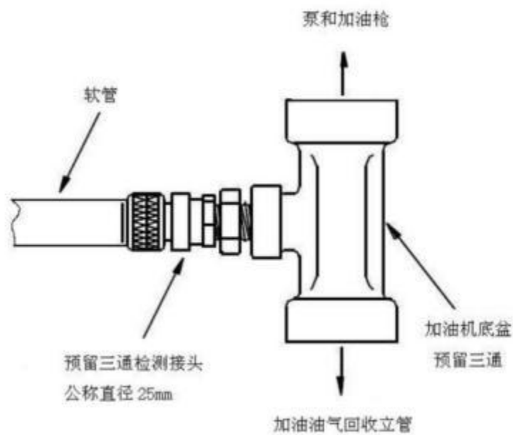
图A.2 三通检测接头示意图
