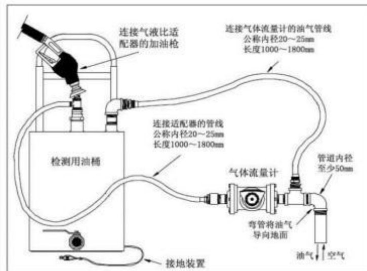
图C.3 气液比检测装置安装示意图
