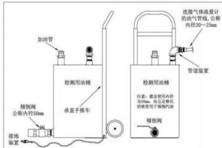
图C.1 气体流量计和气液比适配器安装示意图
