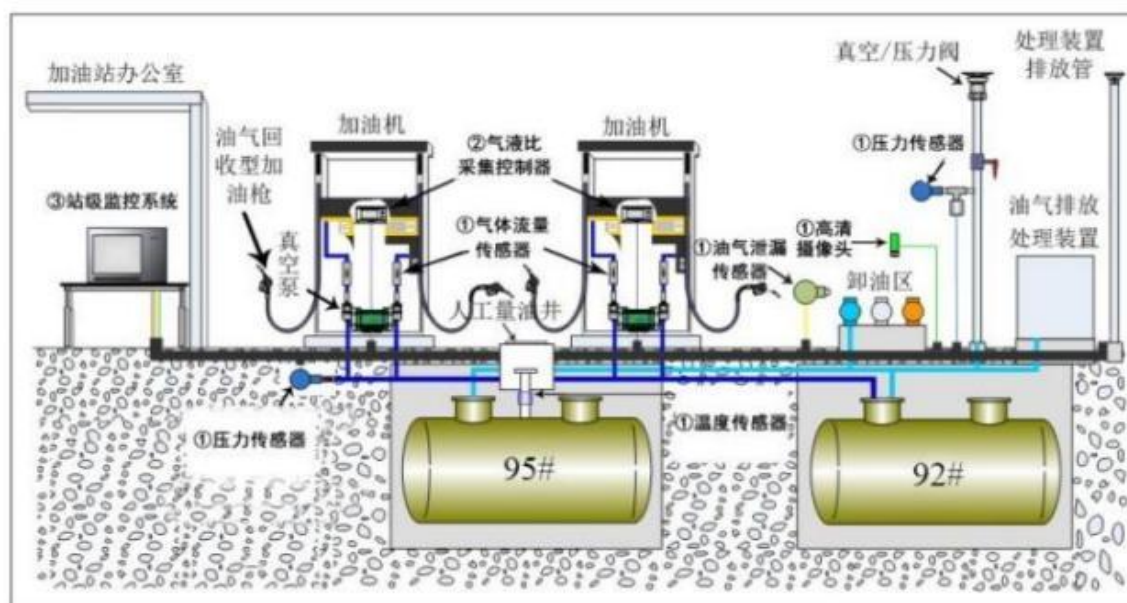
图E.1 在线监控系统
