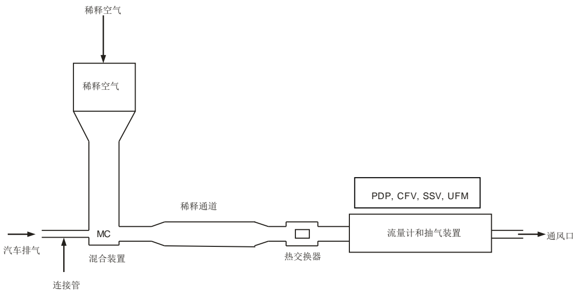
图 CD.3 排气稀释系统
