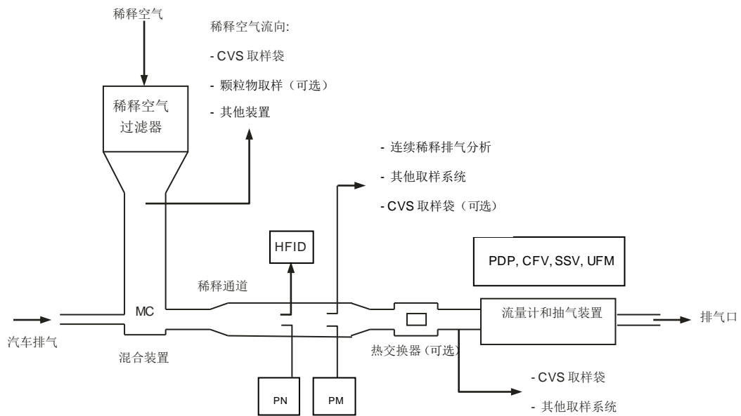
图 CD.9 全流排气稀释系统示意图
