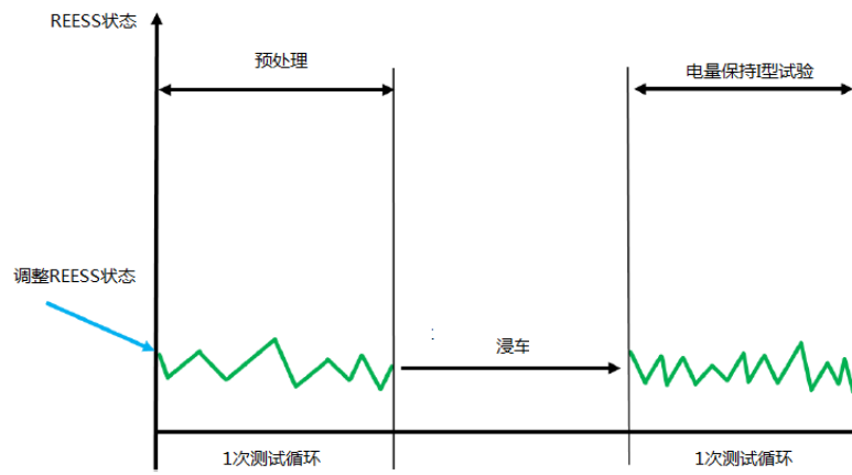
图 RA.5 NOVC-HEV 电量保持 I 型试验
