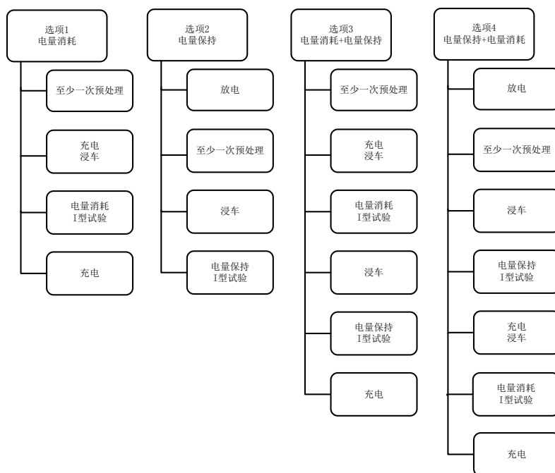
图 R.1 OVC-HEV 测试时可选测试序列
