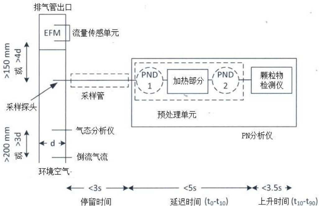
图 DB.1 PN 分析仪原理图
