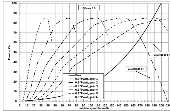
图 CB.2 n_{g_{max}} 为次高档
