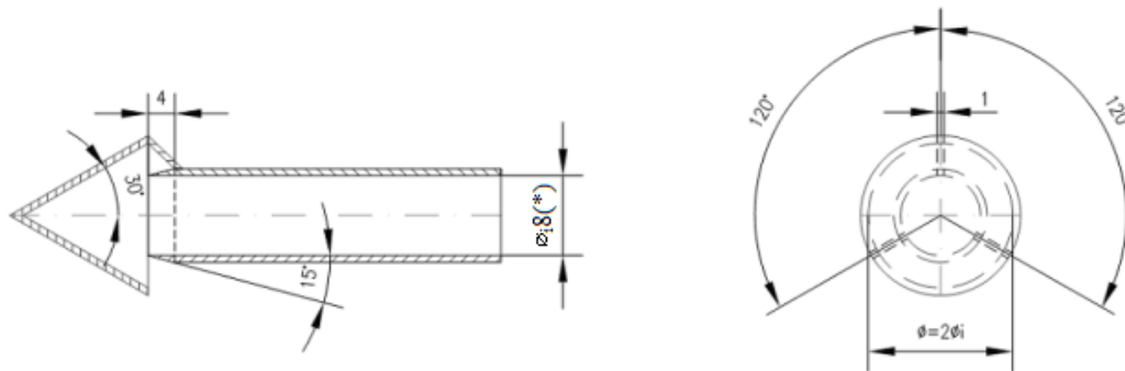
图 CD.11 可选择的颗粒物取样探头示意图
