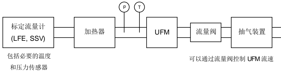
图 CD.8 UFM 标定布置图
