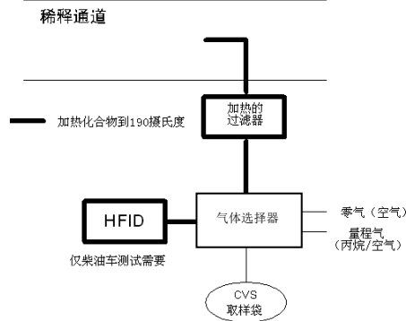
图 CD.10 HFID 取样系统部件示意图
