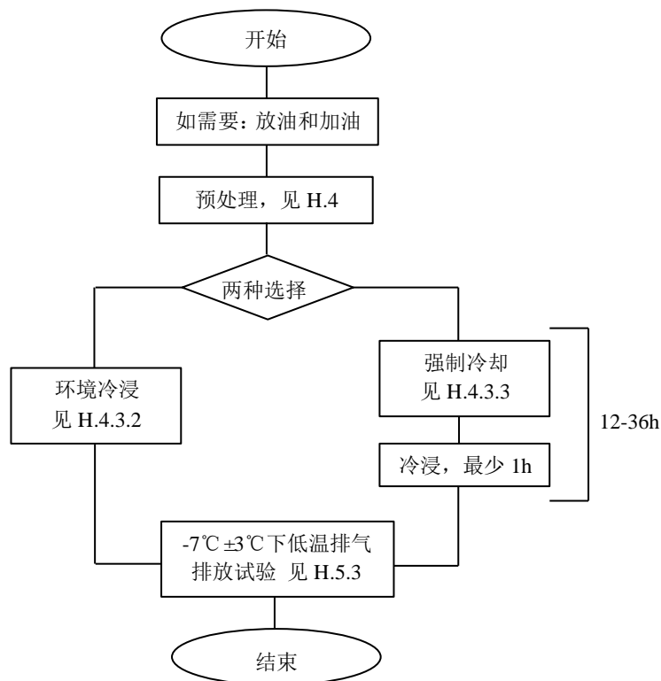
图H.1 低环境温度试验程序
