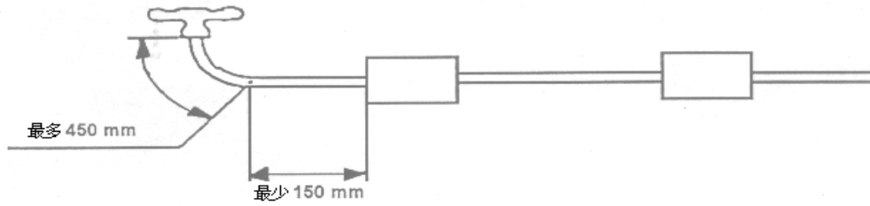
图M.1 背压 - 测量点 (1)
