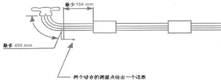
图M.3 背压 - 测量点 (3)
