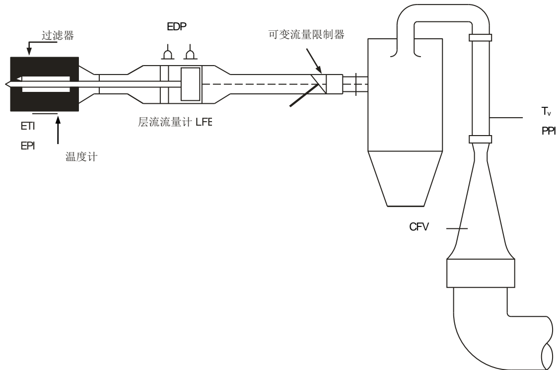
图 CD.7 CFV 标定布置图
