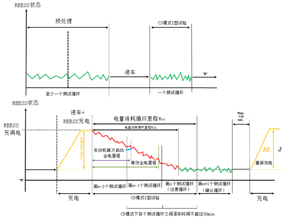
图 RA.4 电量保持 I 型试验和电量消耗 I 型试验
