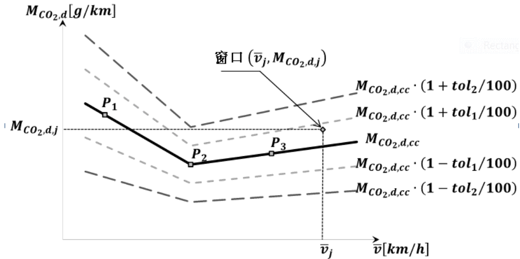
图 DE.3 车辆 CO 2 特性曲线
