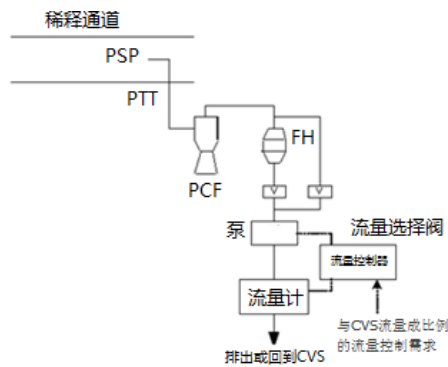
图 CD.12 颗粒物取样系统
