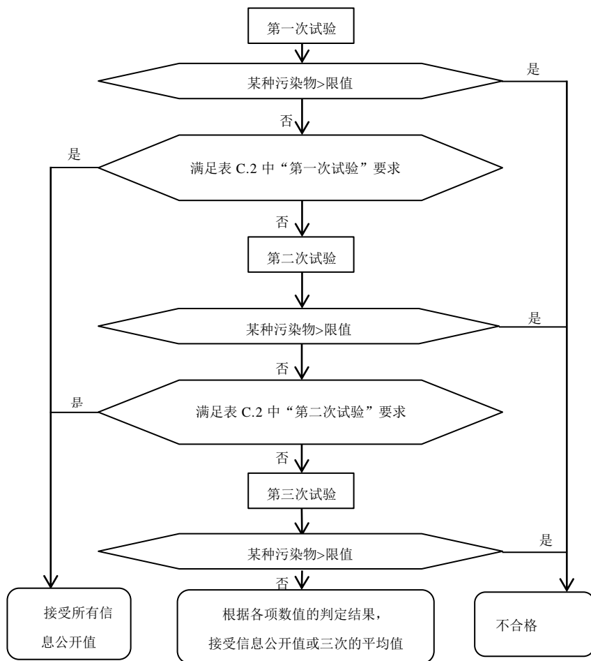
图 C.1 I 型试验流程图
