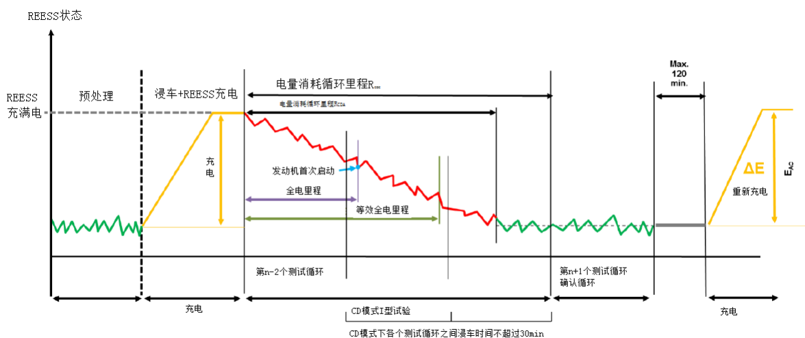
图 RA.1 电量消耗 I 型试验
