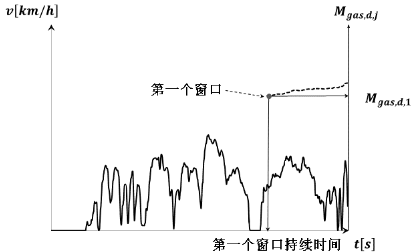
图 DE.1 车速与时间，以及车辆平均排放与时间的关系
