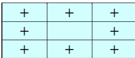
图 CD.1 矩形出风口的测量点示意图
