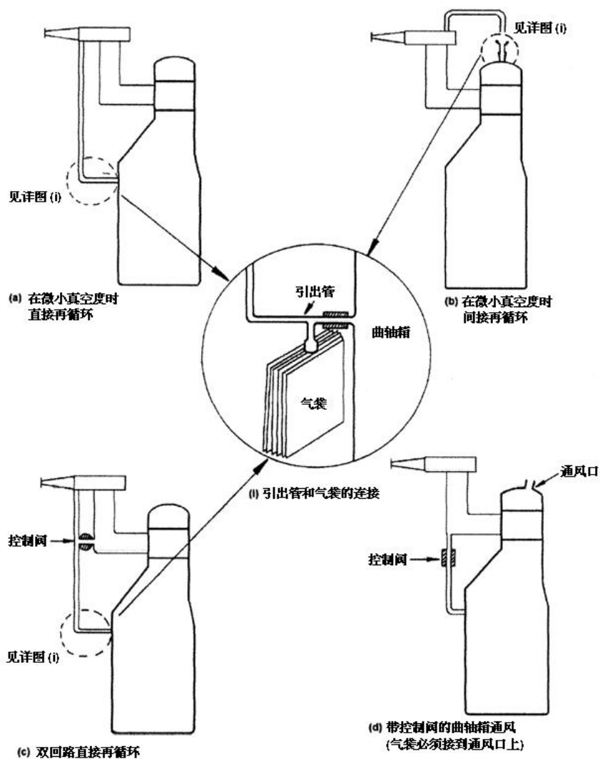
图E.1 III型试验
