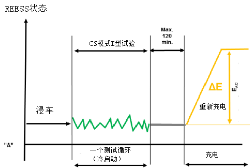
图 RA.3 电量消耗 I 型试验和电量保持 I 型试验
