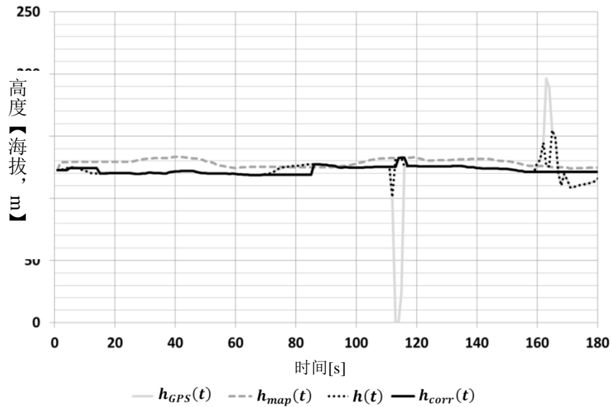
图 DH. 2 数据校正的影响—GPS 测量的海拔高度 h_{GPS}(t) , 等高线地形图提供的海拔高度 h_{map}(t) , 数据校正后的高度 h(t) 和表 DH. 1 中所列数据的校正 h_{corr}(t)
