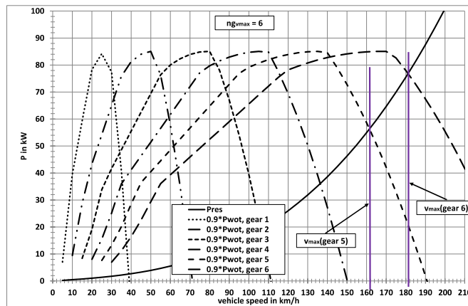
图 CB.1 ng_{vmax} 是最高档
