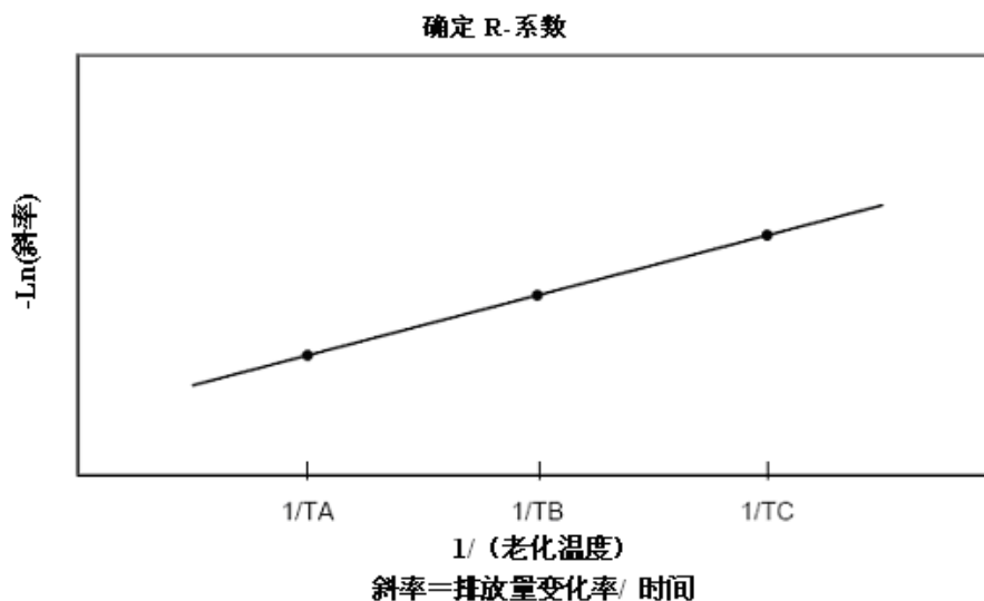
图GA.3 R系数的确定
