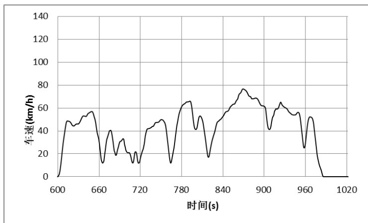
图 CA.2 中速段示意图
