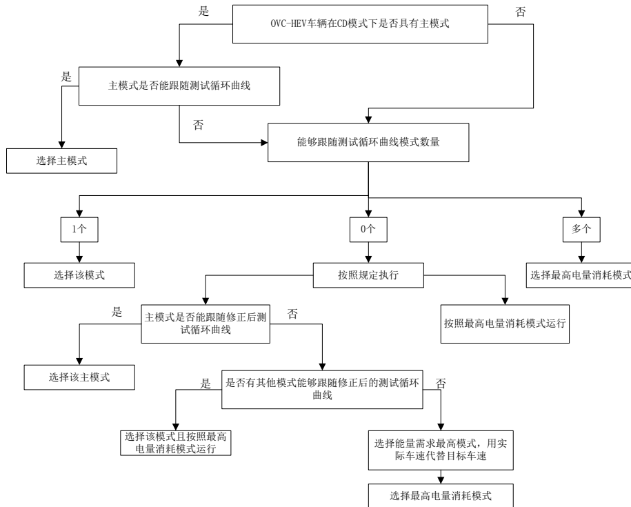
图 RF.1 CD 运行条件下的驾驶模式选择
