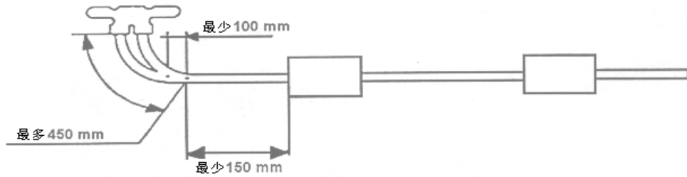
图M.2 背压 - 测量点 (2) (1)
