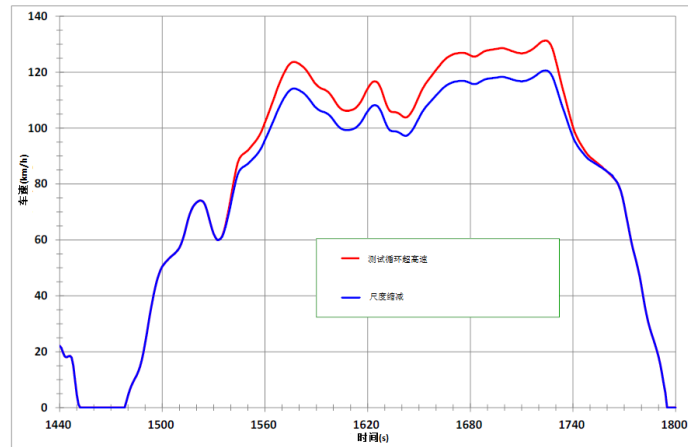
图 CA.5 尺度缩减后的 WLTC 超高速段
