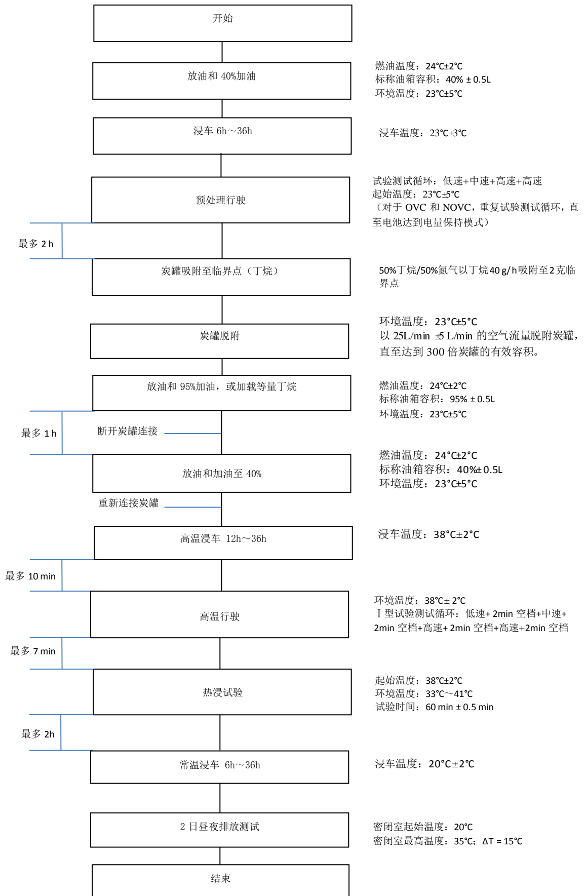
图 F.1b 装备非整体仅控制加油排放炭罐系统 (NIRCO) 汽车的蒸发污染物排放测定规程
