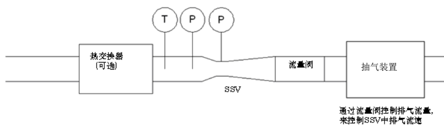
图 CD.4 亚音速管(SSV)示意图
