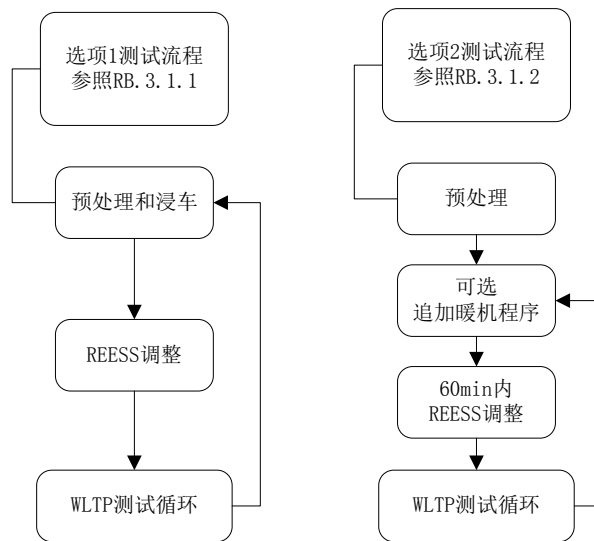
图 RB.1 OVC-HEV 测试流程
