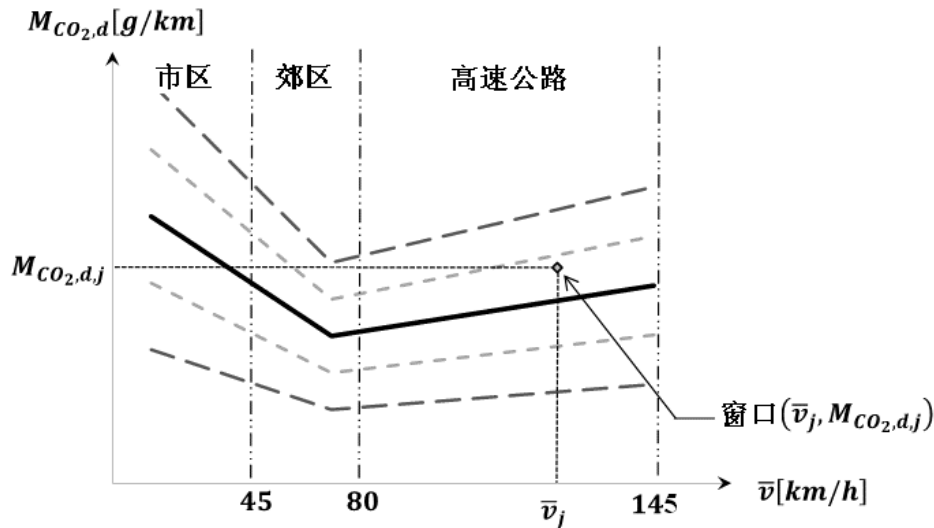
图 DE.4 车辆 CO 2 特性曲线：市区、市郊、高速路段行驶定义
