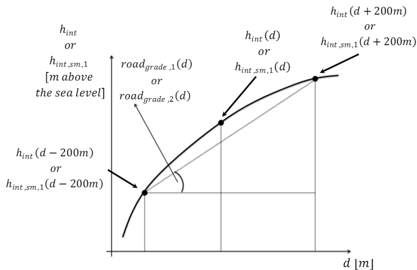
图 DH.1 插值高度信号光滑处理程序示意图
