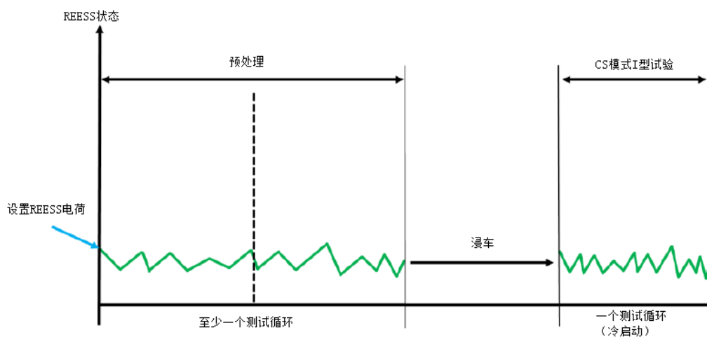
图 RA.2 电量保持 I 型试验
