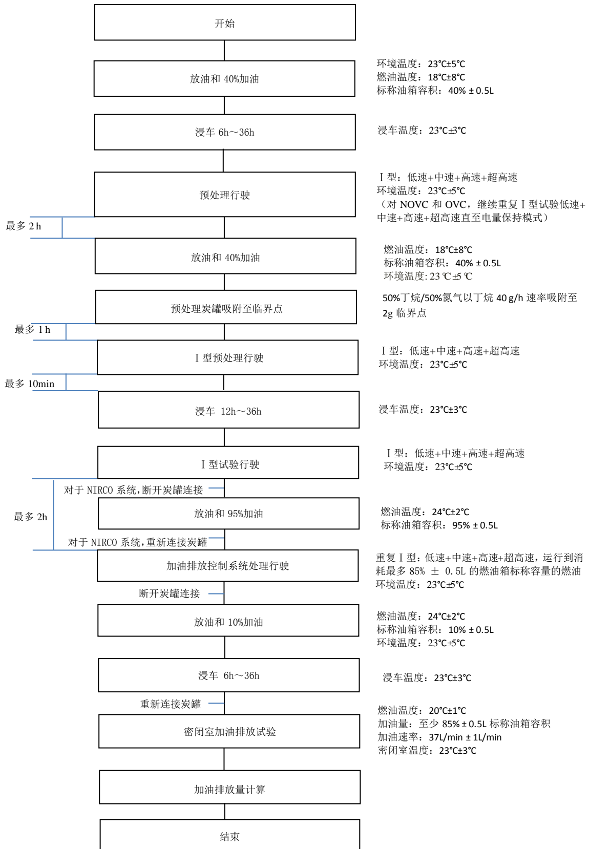
图I.2 非整体或非整体仅控制加油排放（NIRCO）炭罐系统车辆加油过程污染物
