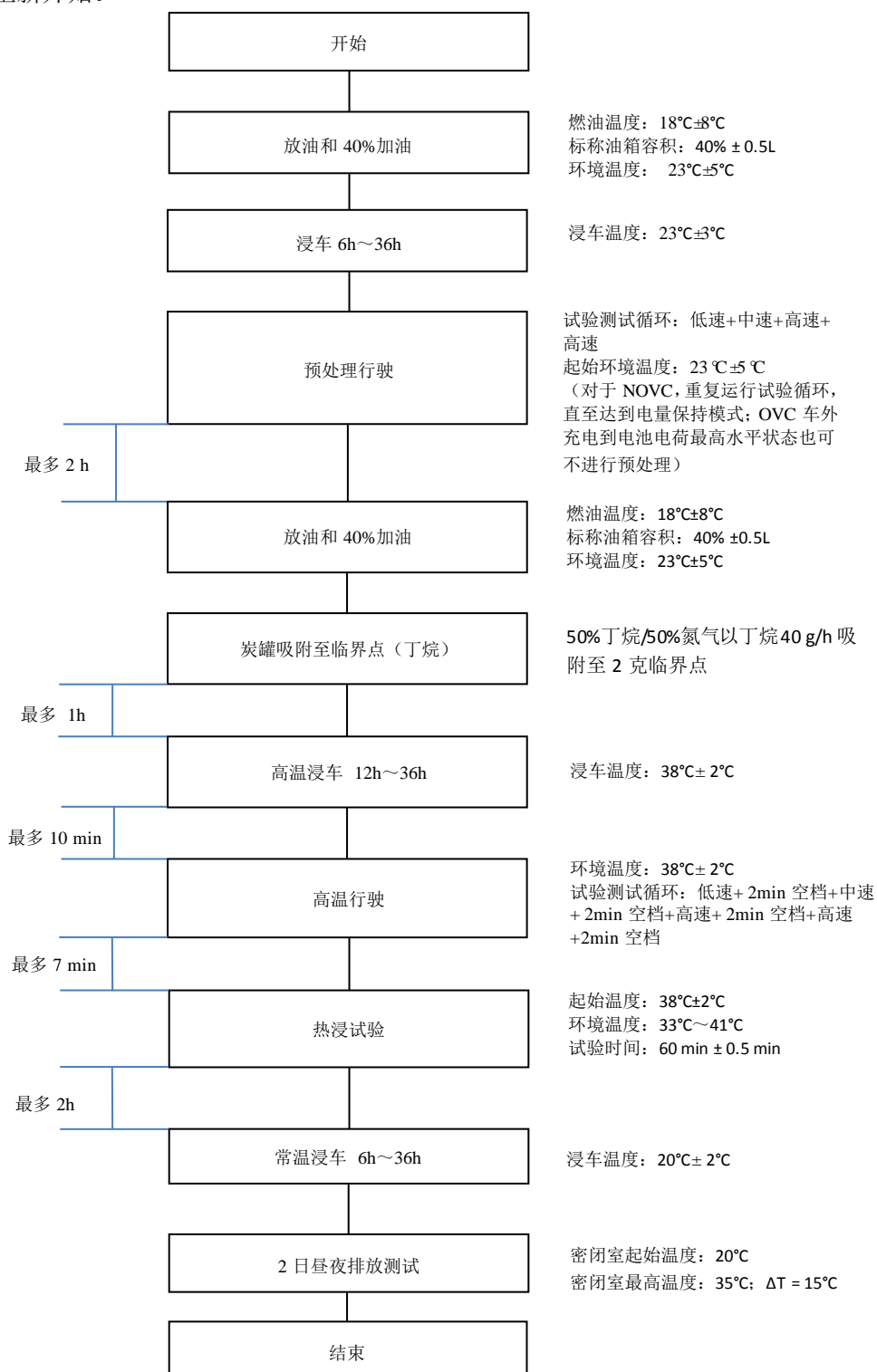
图 F.1a 装备整体炭罐、非整体炭罐系统（NIRCO 除外）汽车的蒸发污染物排放测定规程
