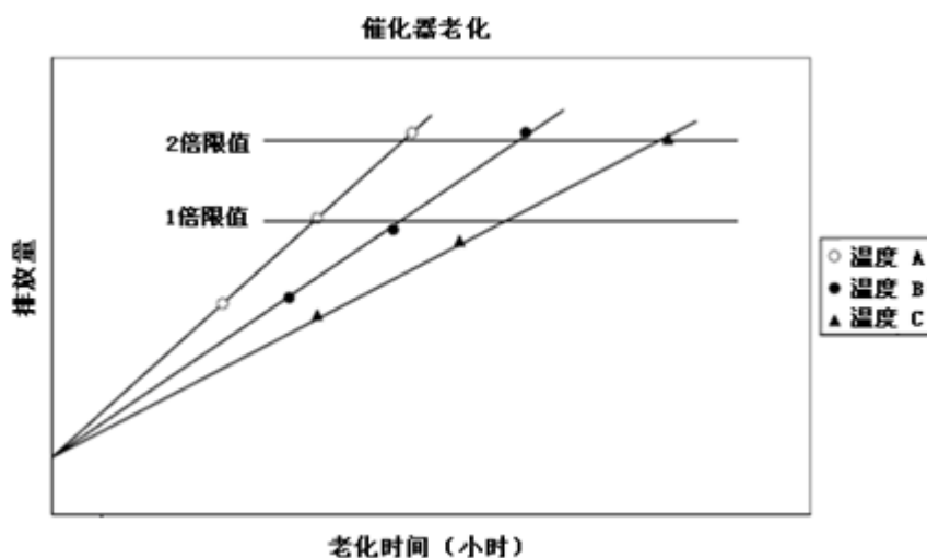
图GA.2 催化剂老化与排放关系
