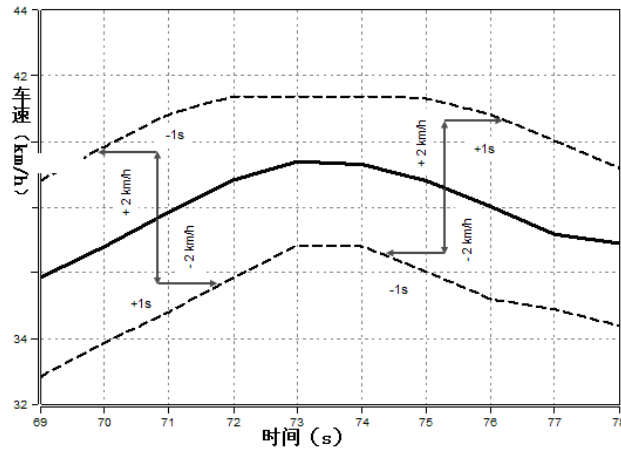
图 C.2 速度曲线公差
