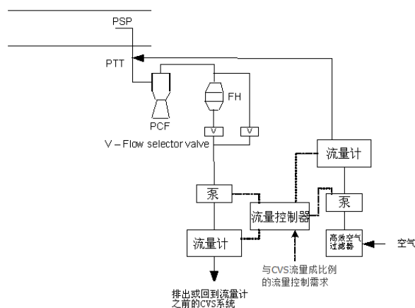
图 CD.13 二级稀释颗粒物取样系统
