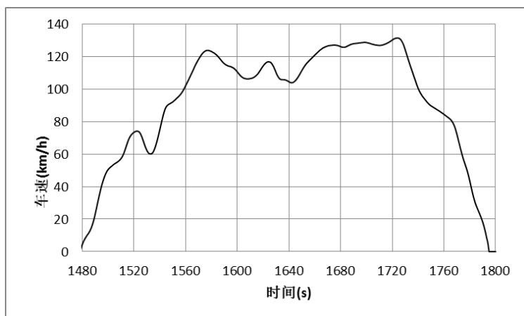
图 CA.4 超高速段示意图
