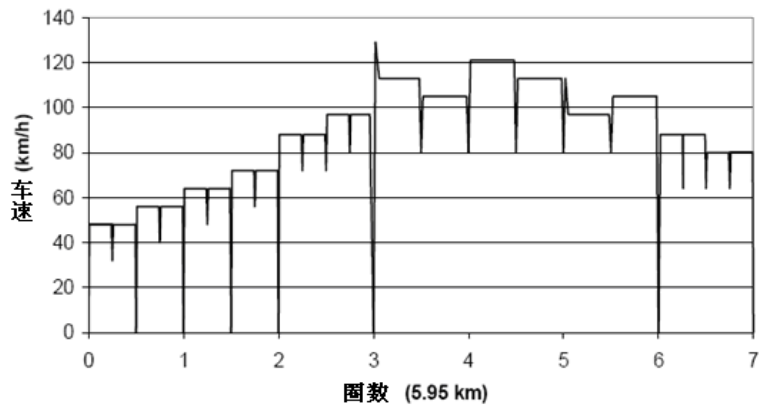
图 GC.1 标准道路循环 (SRC)
