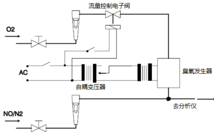
图 CD.15 NO x 转换器效率试验装置
